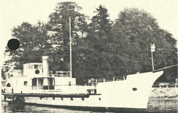
Schauflerraddampfer „Gisela“, Traunsee; erbaut 1870–1872 durch die Werft Floridsdorf bei Wien Foto: Freunde der Stadt Gmunden
